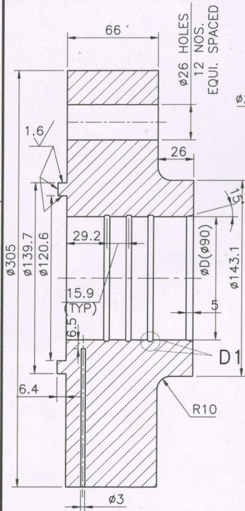
SECTION S1-S1
