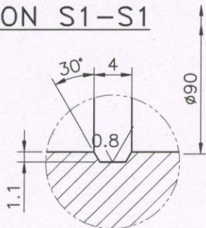
DETAIL D1
